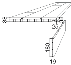
Treppenstufe kompakt 2 x eingeschlagen mit Träger
