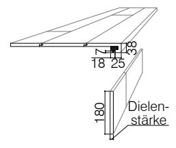
Treppenstufe kompakt 2 x eingeschlagen LED ohne Träger
