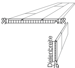
Treppenstufe kompakt 1 x eingeschlagen mit Träger
