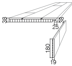
Treppenstufe kompakt 2 x eingeschlagen SPA mit Träger
