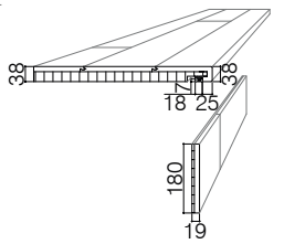
Treppenstufe kompakt 2 x eingeschlagen LED mit Träger
