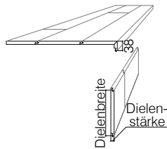
Treppenstufe kompakt 1 x eingeschlagen ohne Träger
