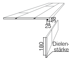
Treppenstufe kompakt 2 x eingeschlagen SPA ohne Träger
