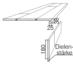
Treppenstufe kompakt 2 x eingeschlagen ohne Träger
