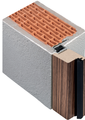
BLENDRAHMEN BM 43/65 in der Laibung mit Blindstock montiert
