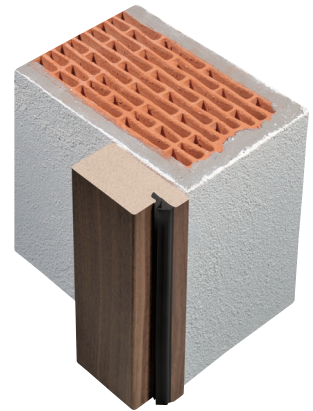
BLENDRAHMEN BM 45 auf der Wand, vor der Laibung montiert
